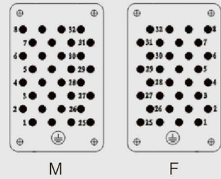
接插针排序
