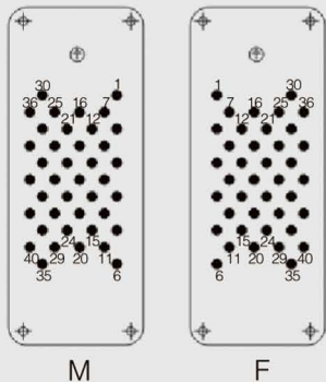
接插针排序
