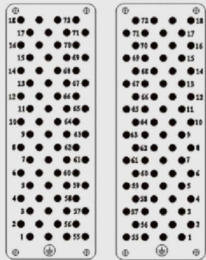
接插针排序
